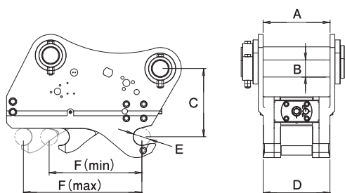
■機械式ワンキヤッチ 仕様図
