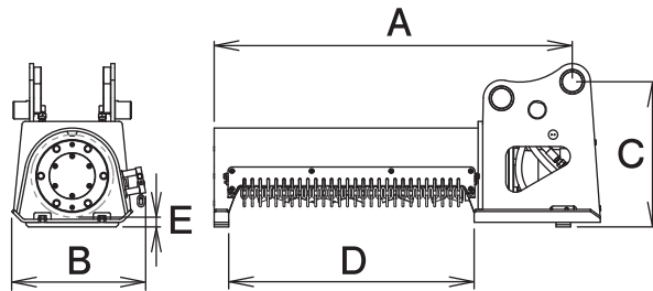
▼首振り(L)タイプ
