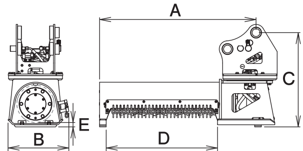
▼リモコン旋回(SC)タイプ
