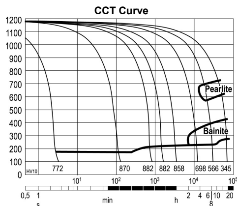
曲線に従って冷却した後の硬さ 焼入れ温度1180℃。
