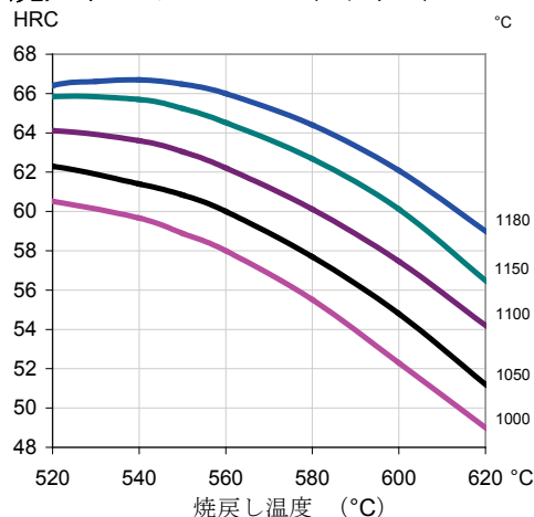
焼入れ、クエンチ、1時間X3回の焼戻し後の硬さ
